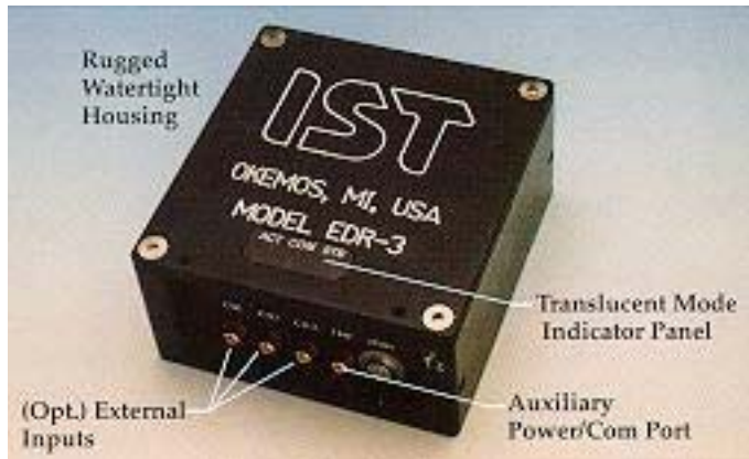
Figure 3. IST EDR-3 Environmental Data Recorder
